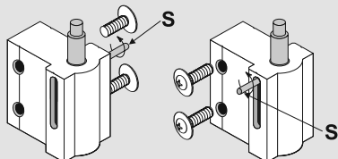
Zawias górny w lewym skrzydle drzwi
