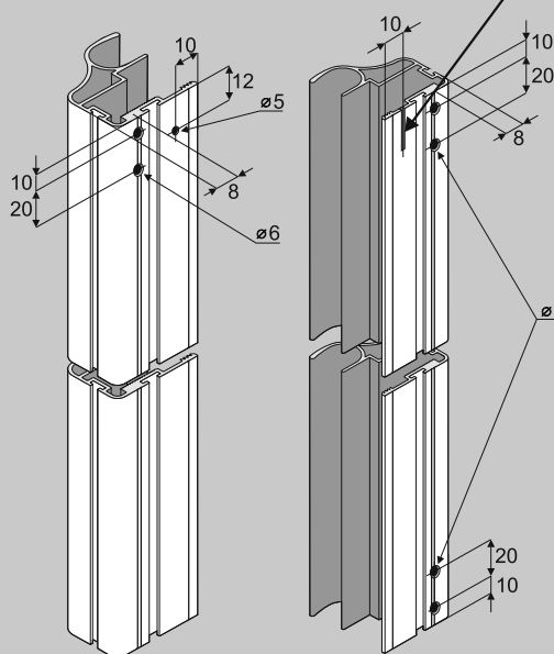
Rozstaw otworów do mocowania zawiasu górnego (B) i zawiasu dolnego (C)
