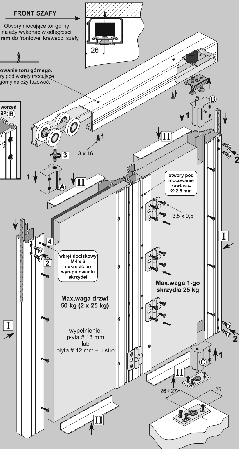
Mocowanie gniazda zawiasu dolnego.
