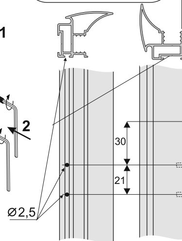
rozmieszczenie otworów do montażu wózka Everest Fox
