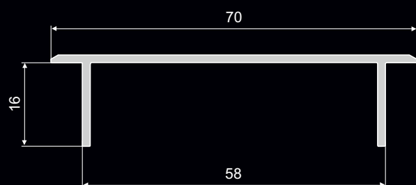
K6 powierzchnia wentylacji поверхность вентиляции 150 cm 2
