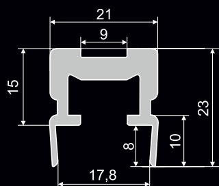
Profil łączący do rury 20×20 Профиль соединительный для трубы 20×20 nr 037 012 05
