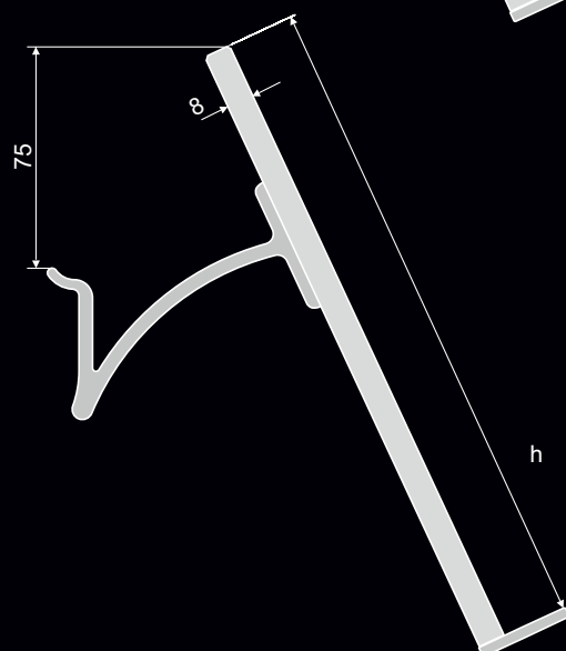
Półka Ekspozycyjna szklana H Стеклянная полка экспозиционная H h 216×300 mm nr 032 059 05
