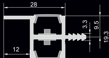
Profil / Профиль ALU LED do wieńca korpusu для окантовки корпуса
