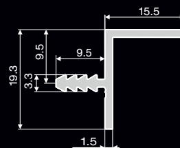
Profil do wieńca korpusu nr 050 019 05 Профиль для окантовки корпуса
