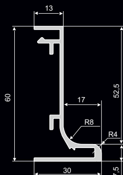
Listwa aluminiowa L
