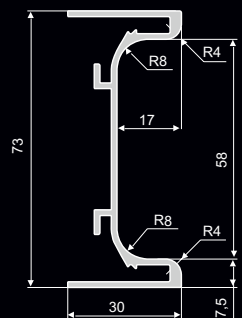
Listwa aluminiowa C
