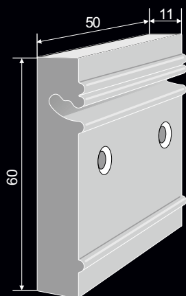
Gniazdo przykręcane Прикручивающийся патрон
